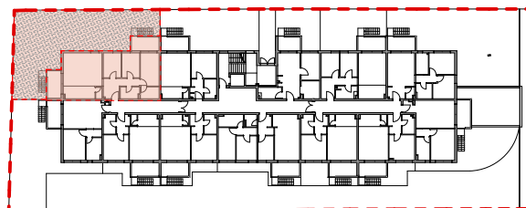
TLOCRT PRIZEMLJA
