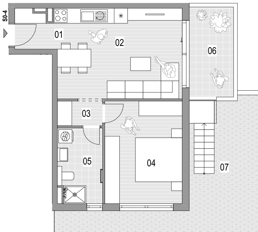
TLOCRT STANA
