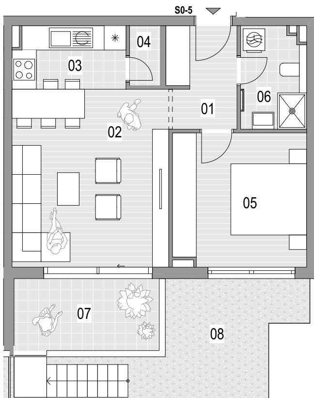
TLOCRT STANA
