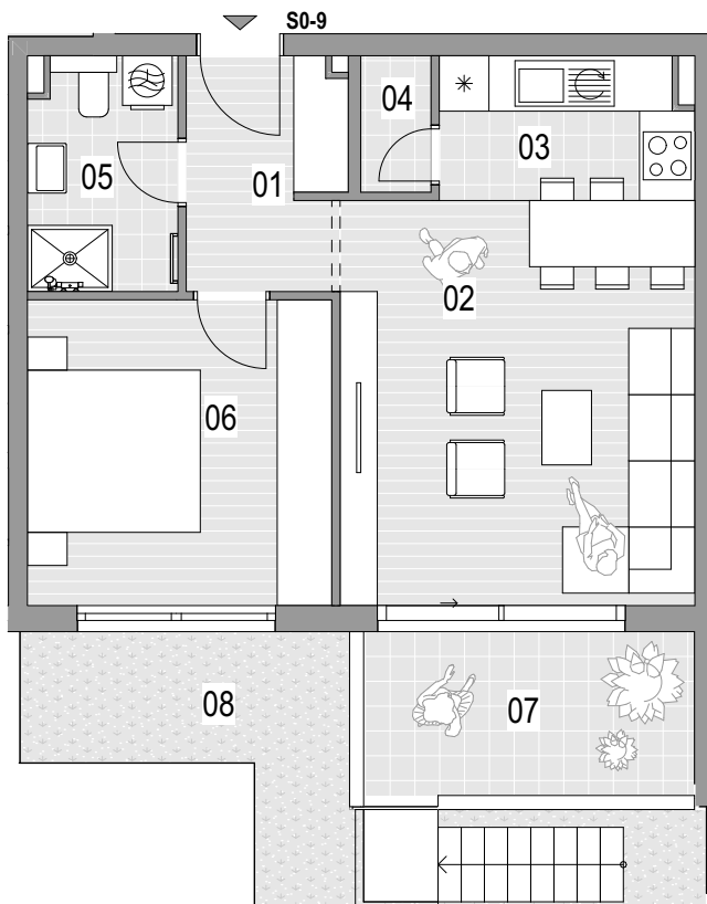
TLOCRT STANA
