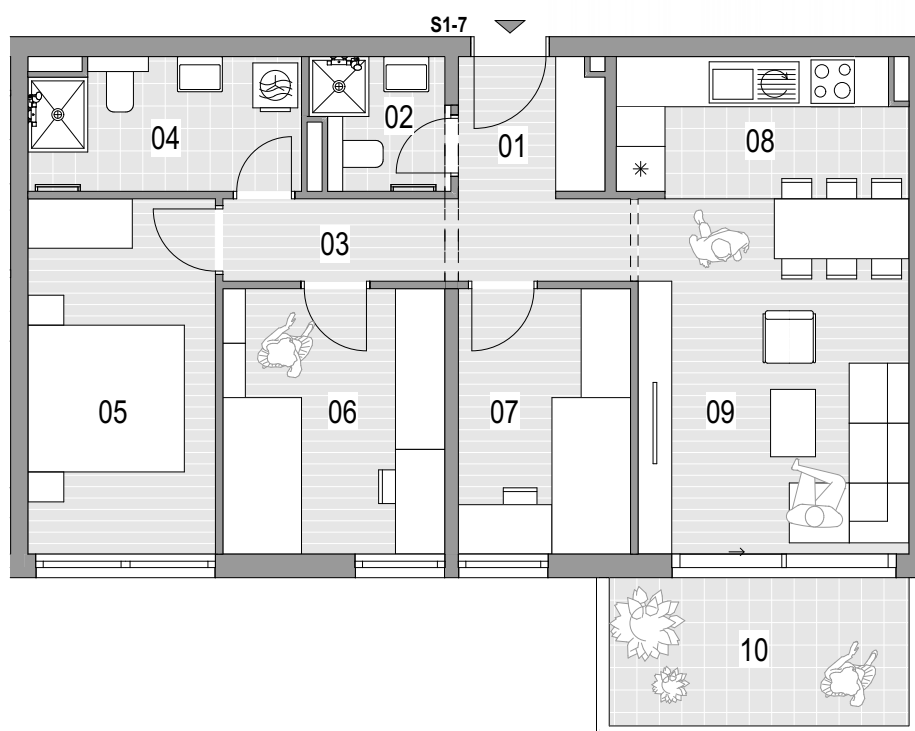
TLOCRT STANA
