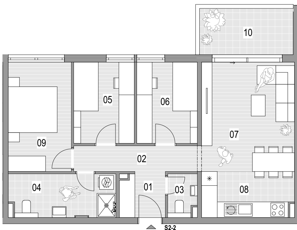
TLOCRT STANA
