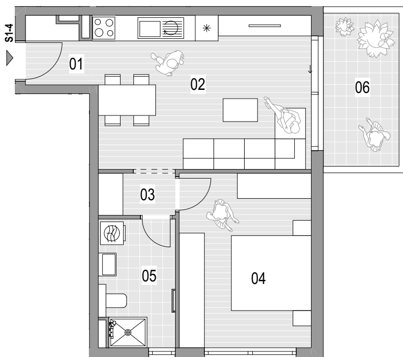
TLOCRT STANA
