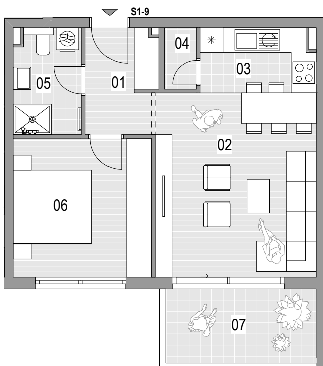
TLOCRT STANA
