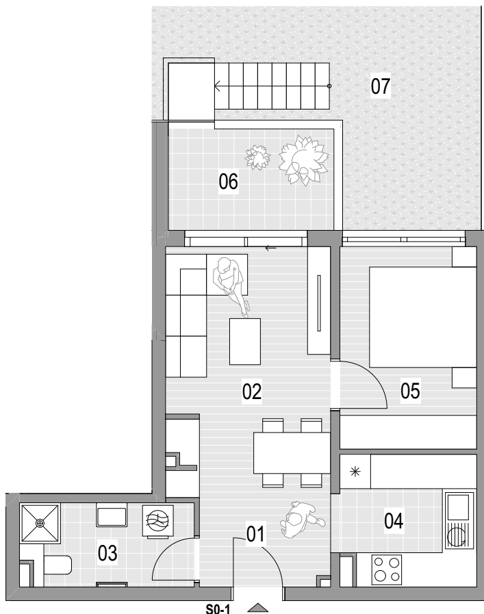
TLOCRT STANA
