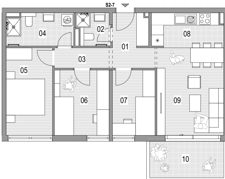
TLOCRT STANA
