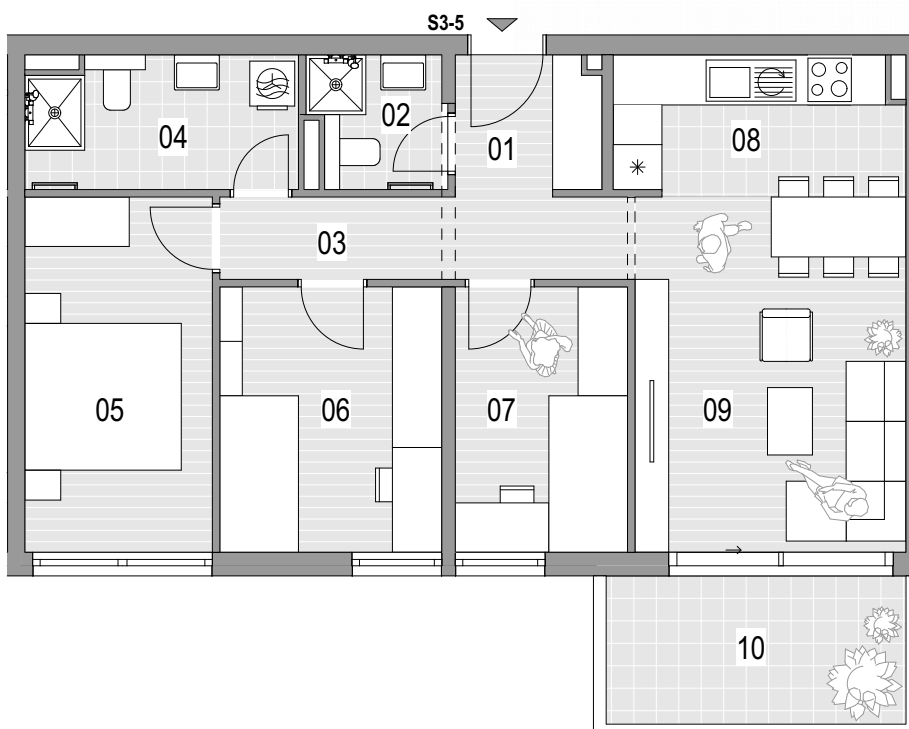
TLOCRT STANA
