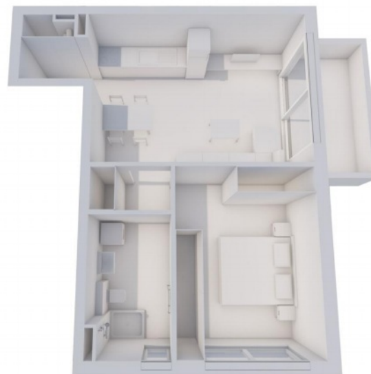
PROSTORNI PRIKAZ
